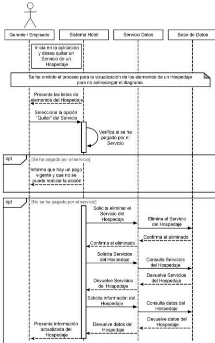
Figura N° 2.78 Diagrama de Secuencia Quitar Servicio de Hospedaje
